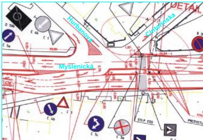
Nové riešenie dopravy pri odbočke na Cintorínsku ul.
