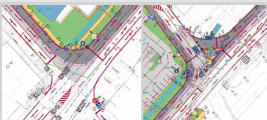
Vľavo detail dopravného riešenia križovatky smer Limbach a vpravo križovatka smerujúca k obchodnému centru.
