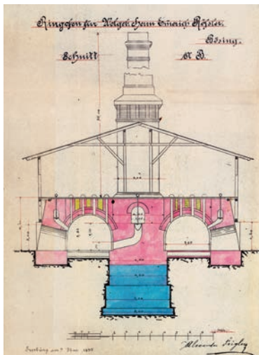
Kruhová pec pre I. Rösslera, rez, A. Feigler, 1895 (zdroj: ŠAB, Archív Modra)
