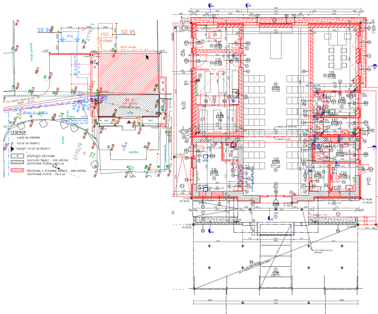
Obr. 1 Časť koordinačnej situácie a pôdorysu 1.NP navrhovaného stavu
