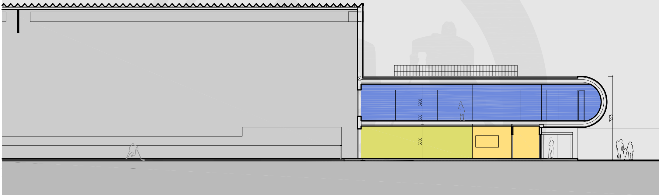
REZ B-B'
