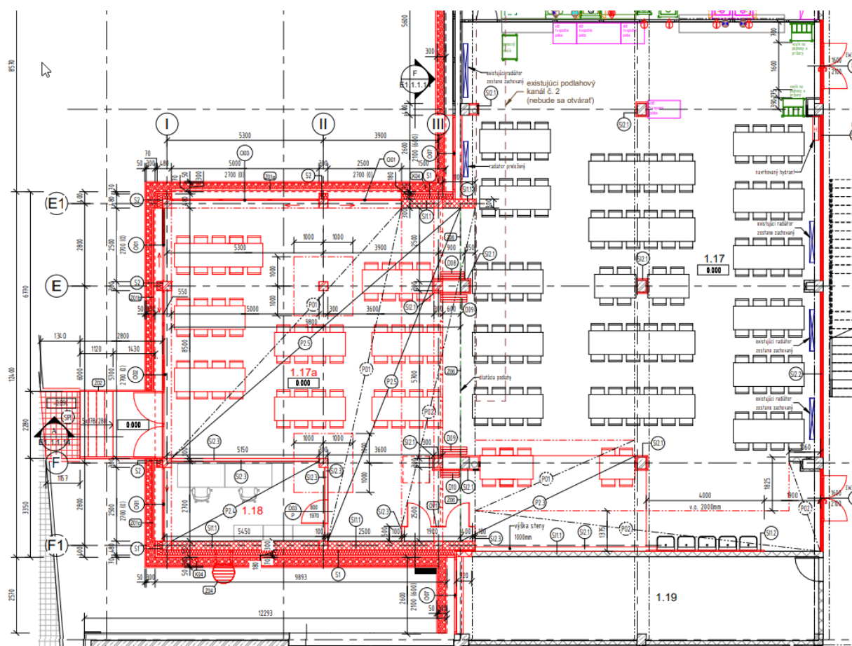
Obr. 1 Navrhovaná prístavba jedálne
