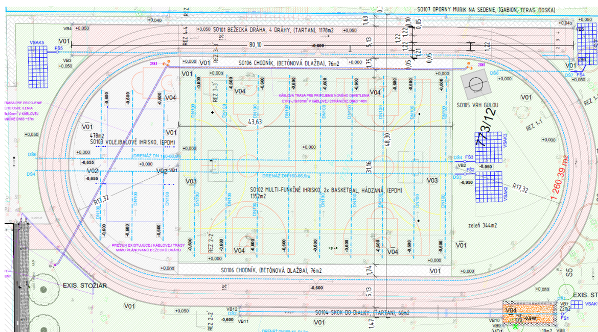
Obr. 3 Navrhovaná modernizácia športoviska
