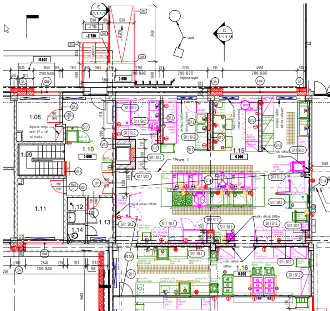
Obr. 2 Navrhovaná rekonštrukcia kuchyne
