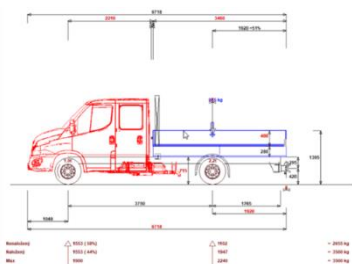
Ilustračný obrázok úžitkového vozidla do 3,5 t
