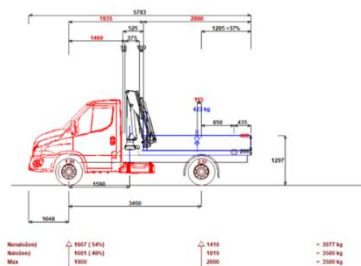
Ilustračný obrázok úžitkového vozidla do 3,5 t
