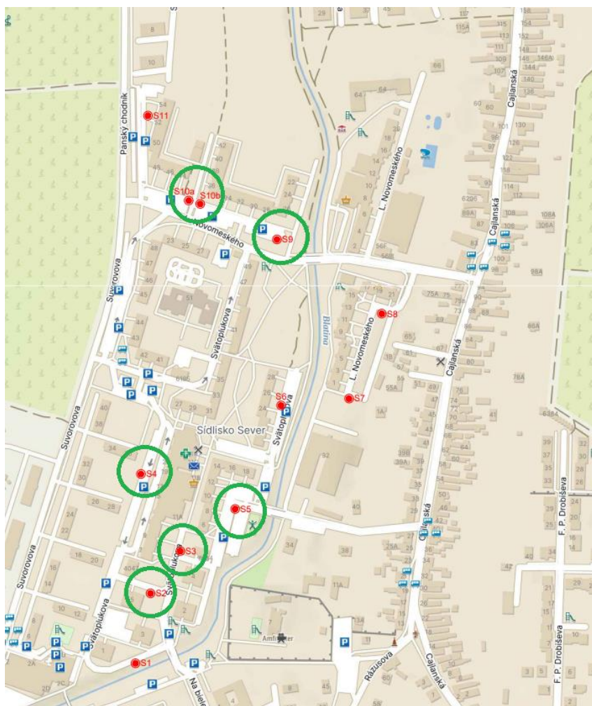
Obr. 9 Situácia rozmiestnenia navrhovaných stojísk
