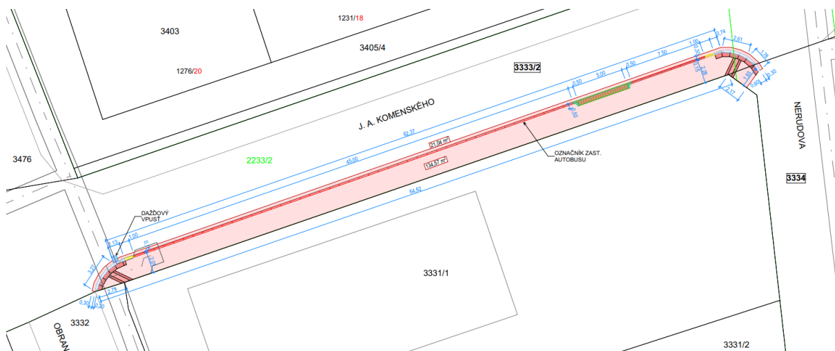
Obr. 6 Navrhovaná rekonštrukcia chodníka Komenského ul. pred ZOS
