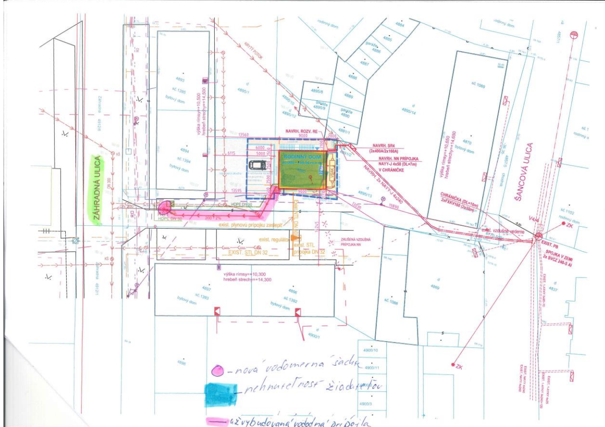
Obr. 1 Koordinačná situácia stavby s vyznačením polohy navrhovanej vodomernej šachty
